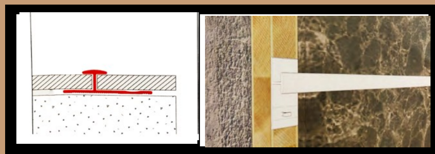
安装示意图 installation diagram
