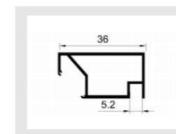
名称: JJ-1996 (四代层板灯) 重量: 0.37kg/m 壁厚:
