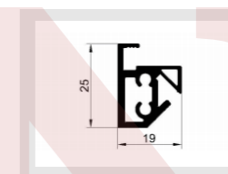
名称: JJ-2037 (三代层板灯) 重量: 0.458kg/m 壁厚: 2.2mm
