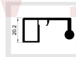
名称: JJ-2011 (20框镂空拉手) 重量: 0.601kg/m 壁厚: 1.8mm
