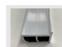
名称: 隐边内嵌拉手 壁厚: 2.8mm 库存颜色: 哑黑、拉丝金
