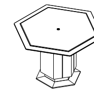
名称 Name 洽谈台 型号 Model LY-006 规格 Size 1200(W)*1040(D)*750(H)mm
