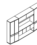
名称 Name 文件柜 型号 Model LY-003 规格 Size 3200(W)*450(D)*2000(H)mm
