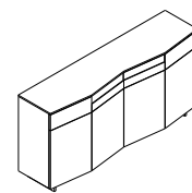
名称 Name 茶水柜 型号 Model LY-004 规格 Size 1600(W)*400(D)*800(H)mm
