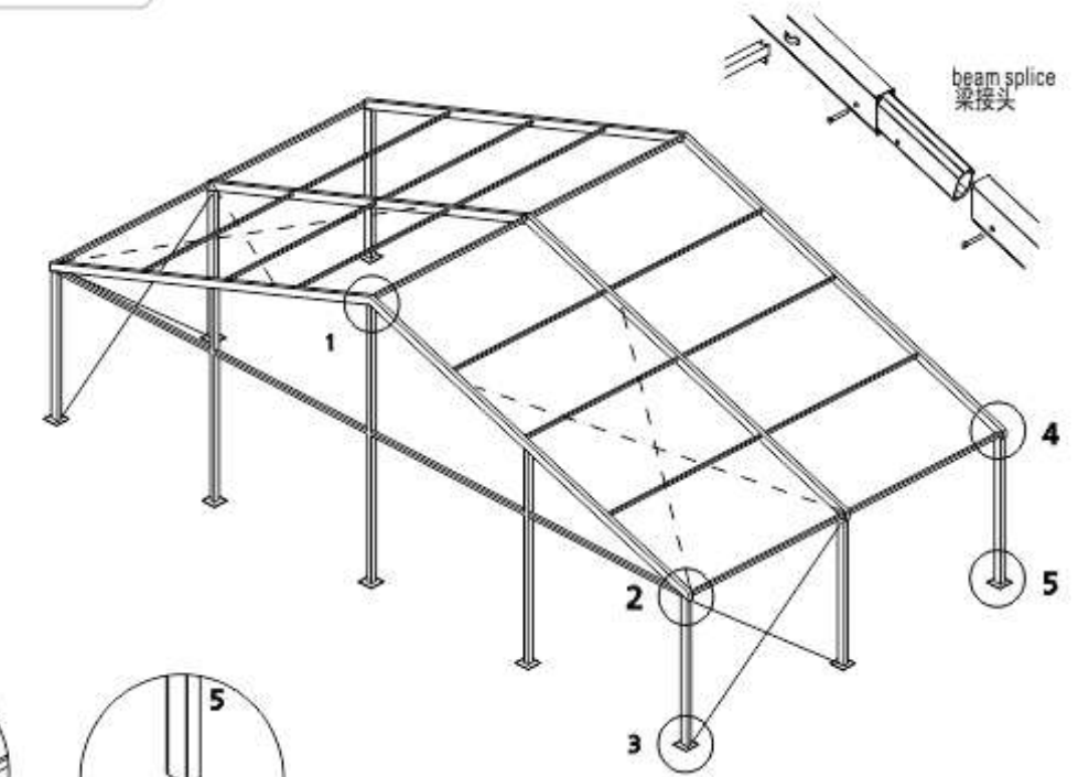
baseplate (field) 底座
