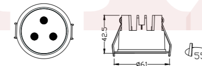
TSD010-55 功率 [Power]: 8W 材质 [Material]: Die-cast aluminum 开孔 [Cut Hole]: Φ55mm
