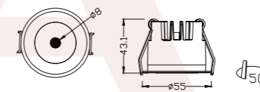
TSD010-50 功率 [Power]: 4W 材质 [Material]: Die-cast aluminum 开孔 [Cut Hole]: Φ50mm
