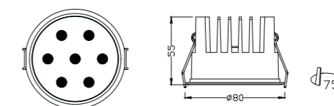
TSD010-75 功率 [Power]: 15W 材质 [Material]: Die-cast aluminum 开孔 [Cut Hole]: Φ75mm
