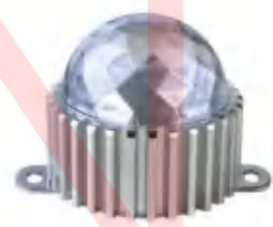
DQ-45404 3-5W 灯体材质: 铝材 工作电压: DC24V LED 光色: R/Y/B/G/W/WW/RGB
