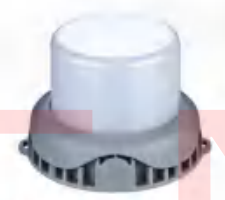
DQ-45402 3-5W 灯体材质: 铝材 工作电压: DC24V LED 光色: R/Y/B/G/W/WW/RGB
